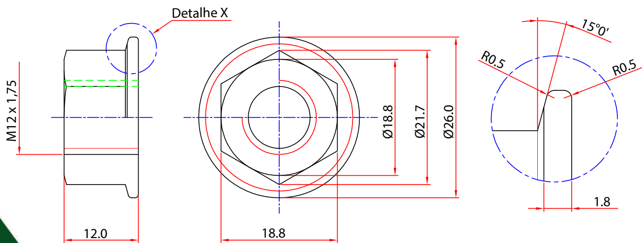
Detalhe X - Escala 5:1
